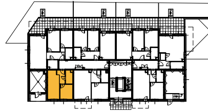
Schemat budynku Lokalizacja mieszkania
